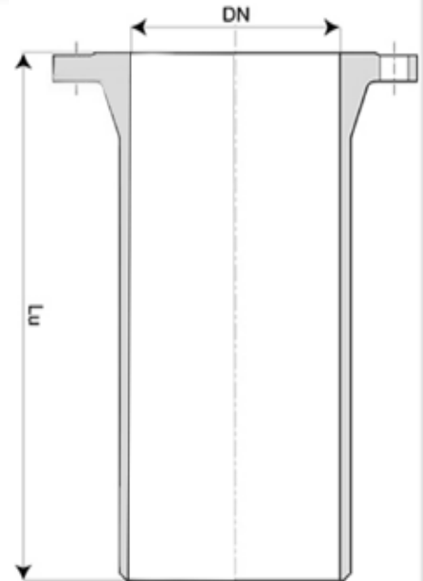
Niple Brida-Espiga
